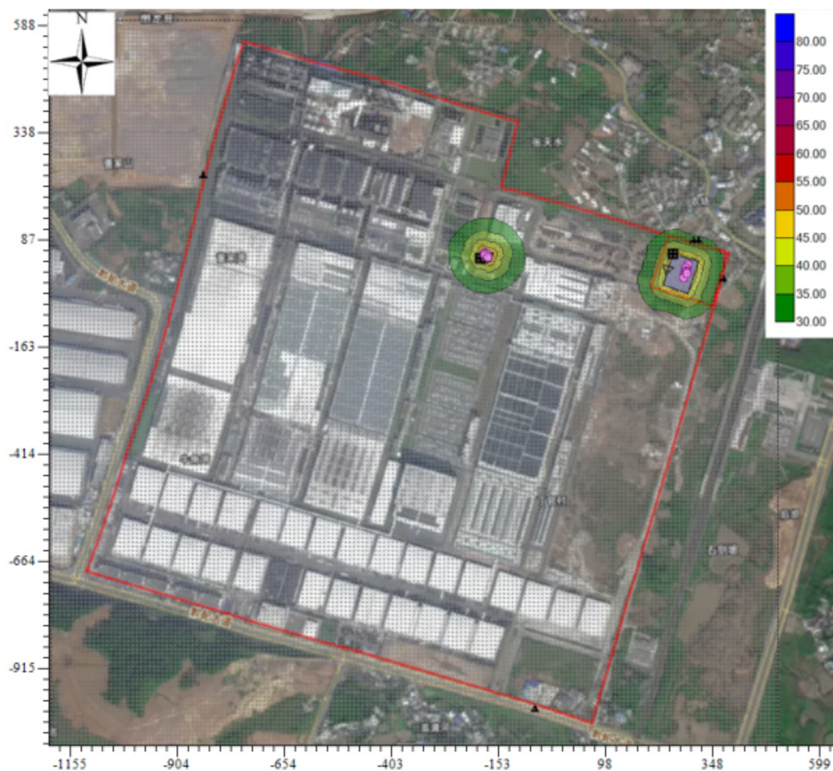
图 4.4-1 运营期等声值线图
