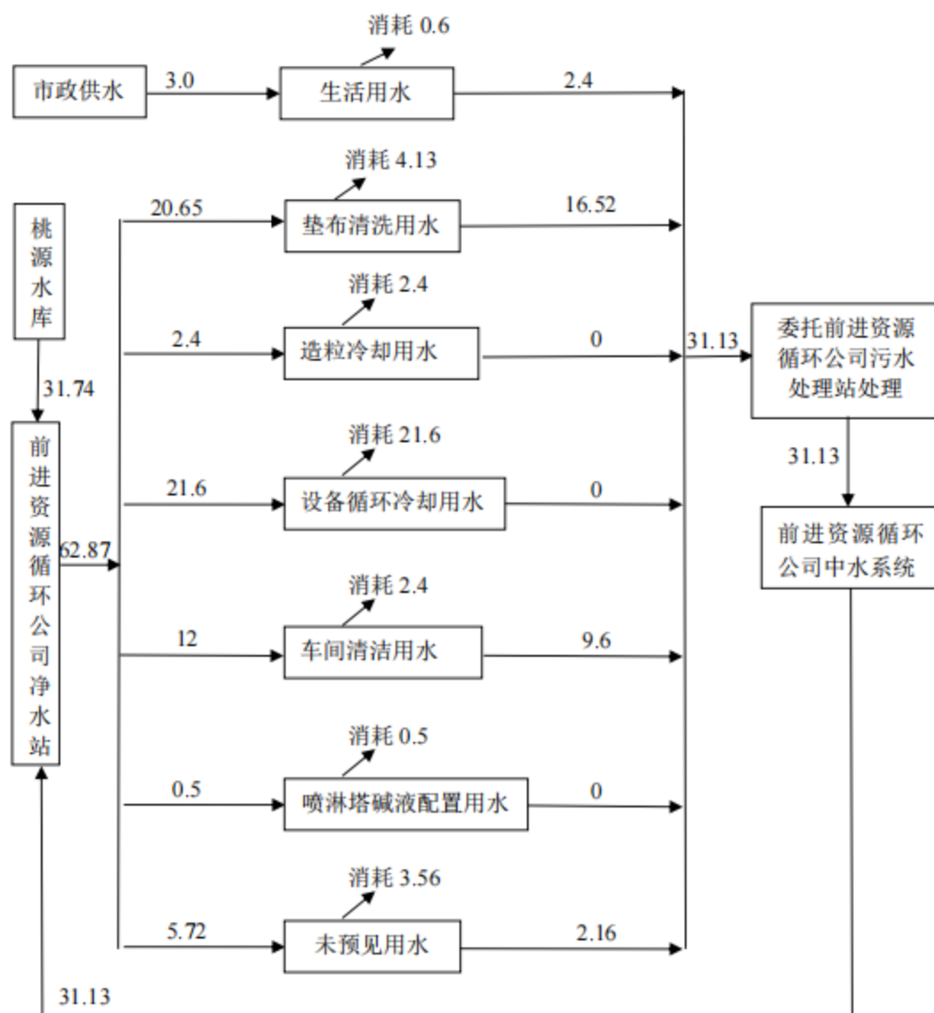
图 2.2-1 本项目水平衡图 (单位 \text{m}^3/\text{d} )
