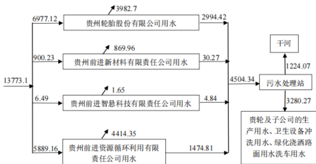
图 2.2-2 项目建成后全厂水平衡图（单位 \text{m}^3/\text{d} ）
