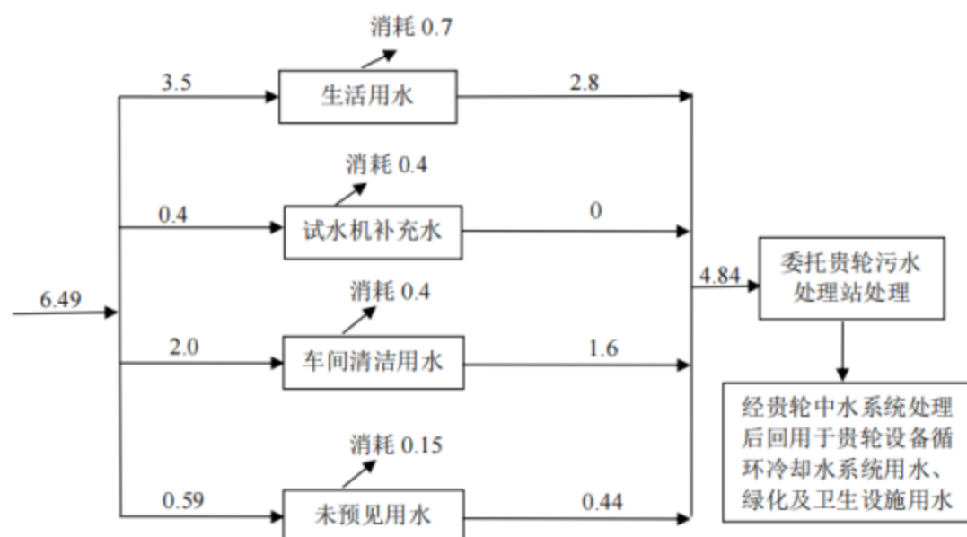
图 2.1-3 现有项目水平衡图 (单位 \text{m}^3/\text{d} )
